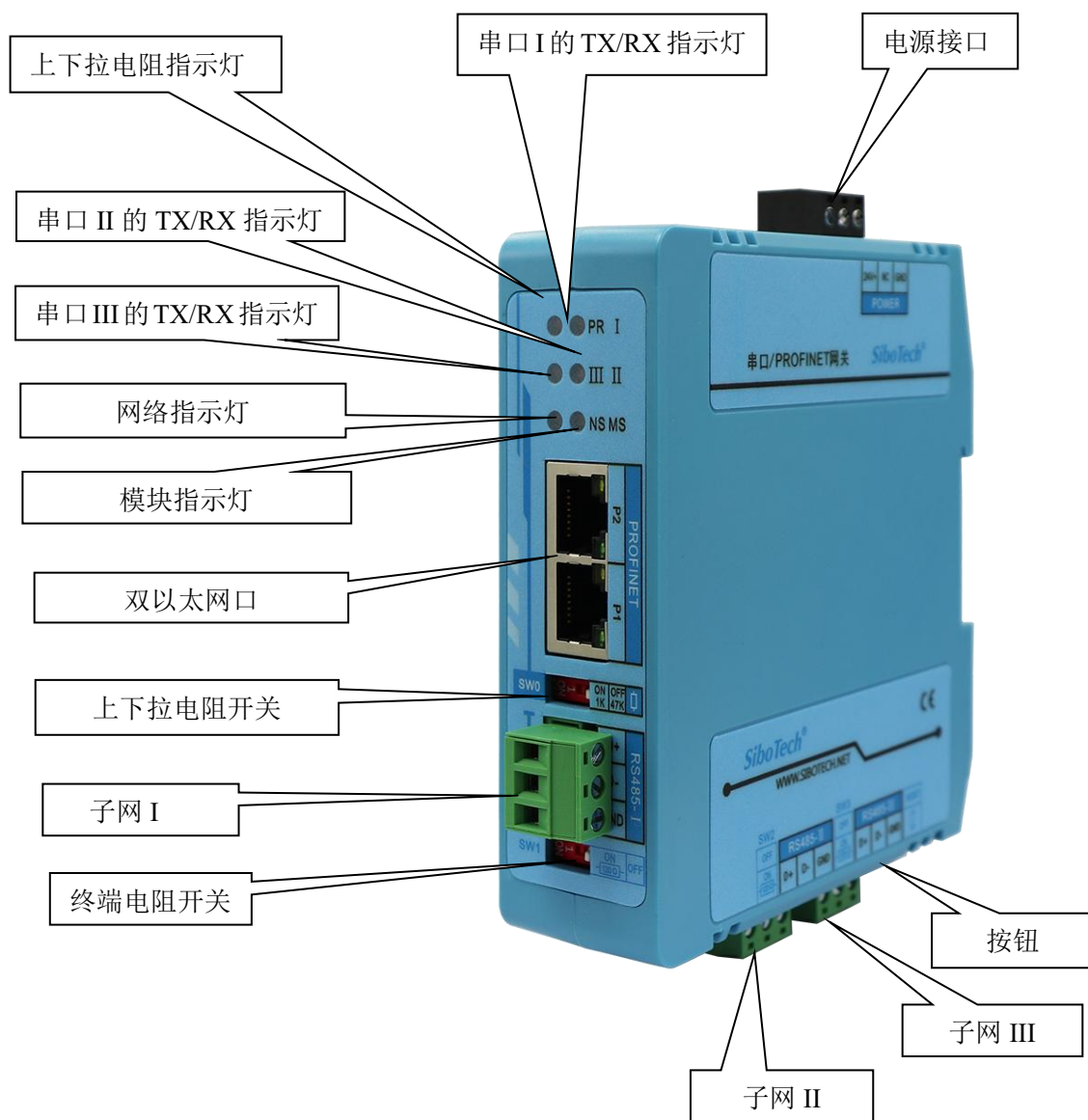
图 1 产品外观
